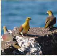
Treron sieboldii <SPRING> <SUMMER> <FALL>
